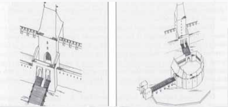
Rekonštrukčné kresby Jany Husárovej znázorňujúce preklenutie priekopy pred Michalskou bránou tzv. padacím mostmi na začiatku 15. storočia (vľavo) a v 2. polovici 15. storočia (vpravo) po postavení barbakánu.
